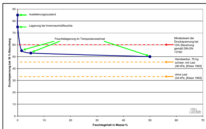
Druckspannung bei 10 % Stauchung in Abhängigkeit vom Feuchtegehalt
